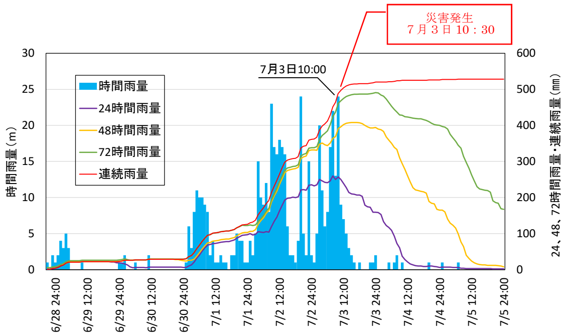
図 1-4 災害発生までの降雨の状況（熱海雨量観測所）
