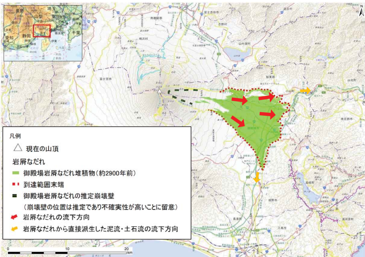
図 2.3-2 御殿場岩層なだれ堆積物の分布と推定崩壊壁
