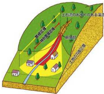
《土石流》
