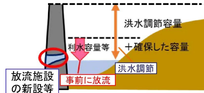
洪水発生前に、利水容量の一部を事前に放流し、洪水調節に活用
