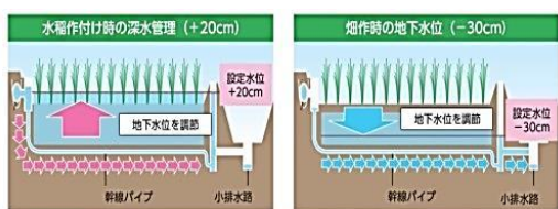
地下水水位の自在の調整が可能 地下水水位制御システム
