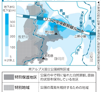
地下水位(計算上)予測値低下量(トンネル掘削完了20年後)
