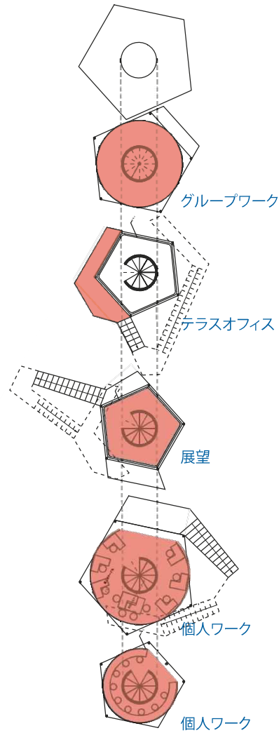
平面図 S=1/200(A1)
