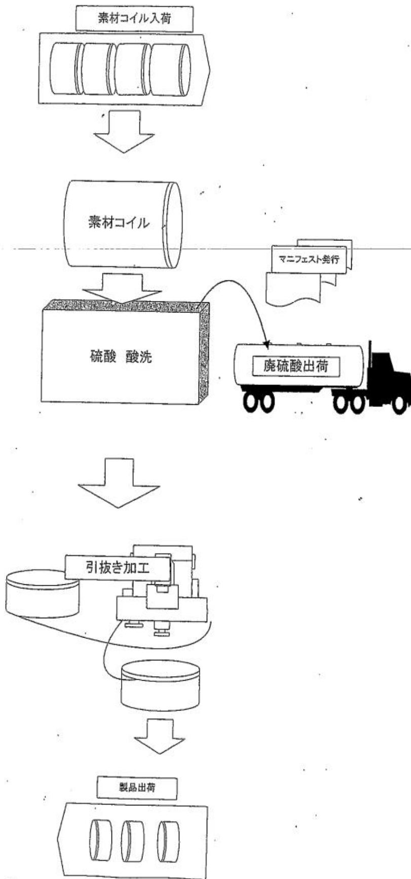
図1 特別管理産業廃棄物の発生工程
