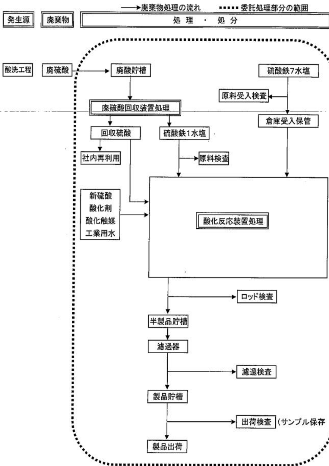
図3-2 特別管理産業廃棄物処理フロー図2
