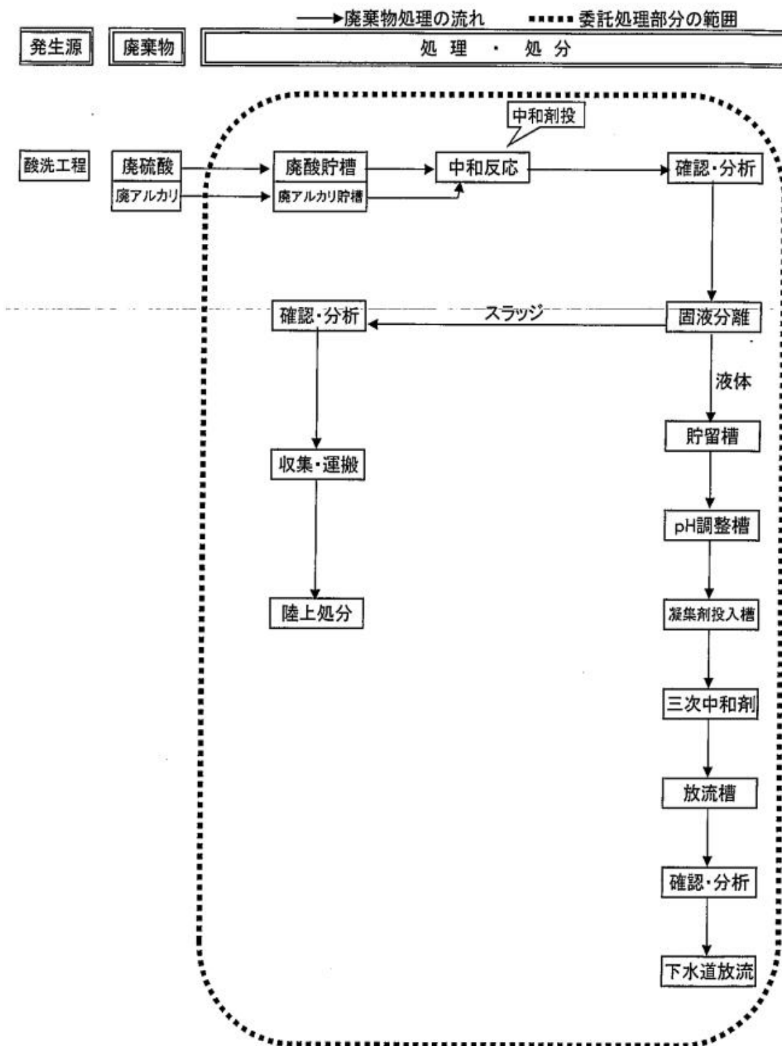
図3-1 特別管理産業廃棄物処理フロー図1
