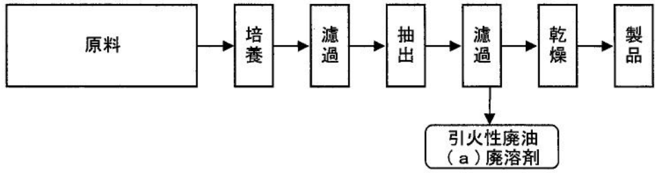
図1 酵素剤製造工程フローシート
