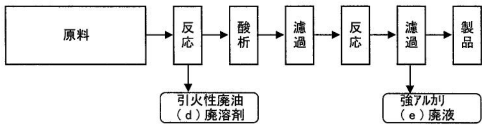
図3 2-クロル-6-メルカプト安息香酸-2ナトリウム塩製造工程フローシート
