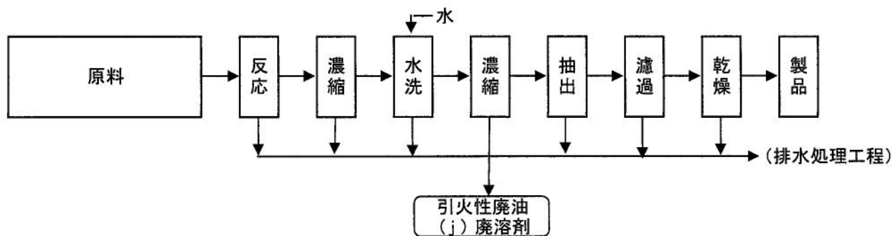
図6 N,N'-(2,2'-ジエチル-6,6'-ジメチル-4,4'-メチレンジフェニル)ビスアレイミド製造工程フローシート
