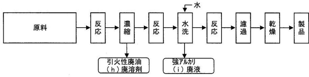
図5 カルシウム-3-オキシド-5-オキシド-4-プロピル-2-オキシド-3-シクロヘキセンカルボキシルト製造工程フローシート
