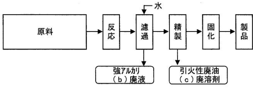
図2 シラン化合物製造工程フローシート
