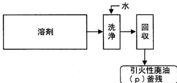
図8 製造設備洗浄工程フローシート
