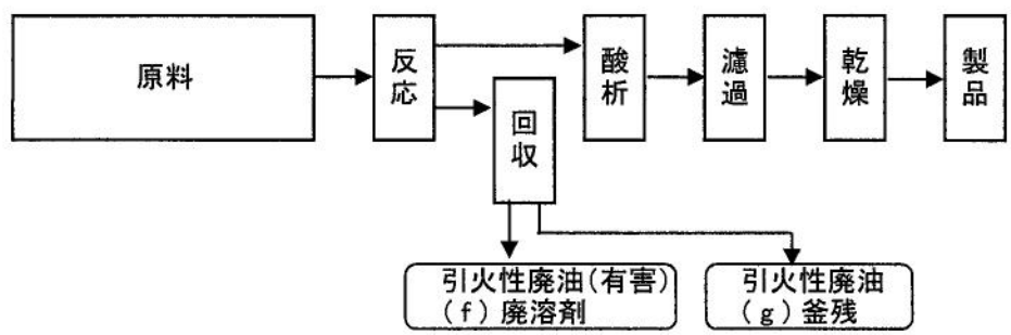
図4 2,6-ジメトキシ安息香酸製造工程フローシート
