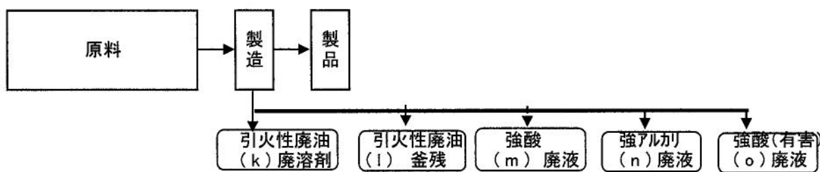
図7 その他の化成品製造工程フローシート
