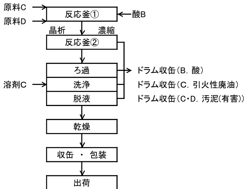
図2 液晶ディスプレイ用感光性化学品製造フローシート
