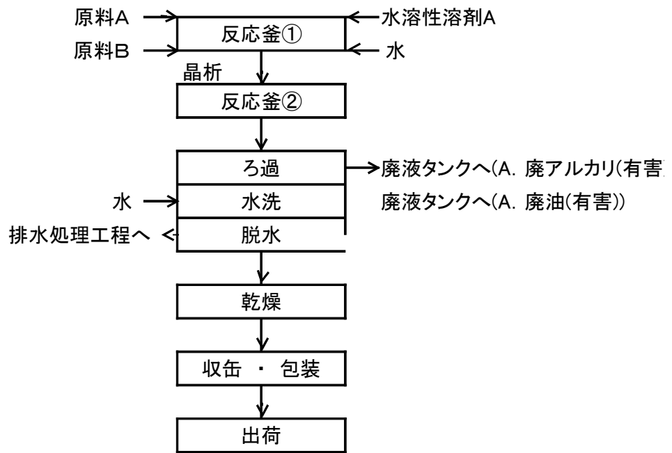
図1 半導体用感光性化学品製造フローシート
