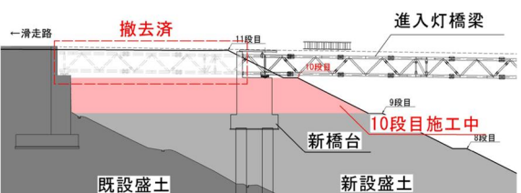
RESA 横断面図(上部)(令和8年9月末時点)
