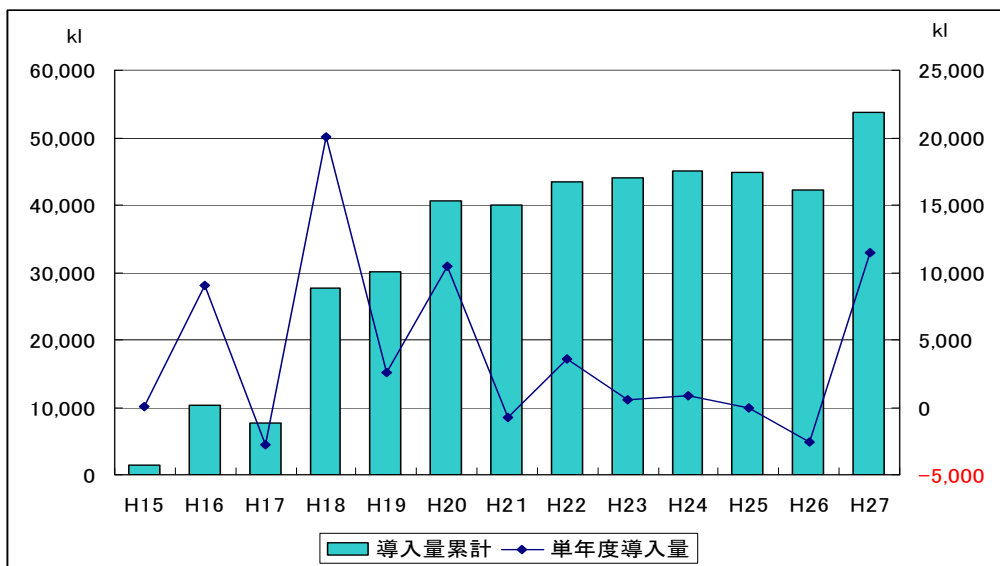
(図表 17) 本県のバイオマス熱利用の推移
