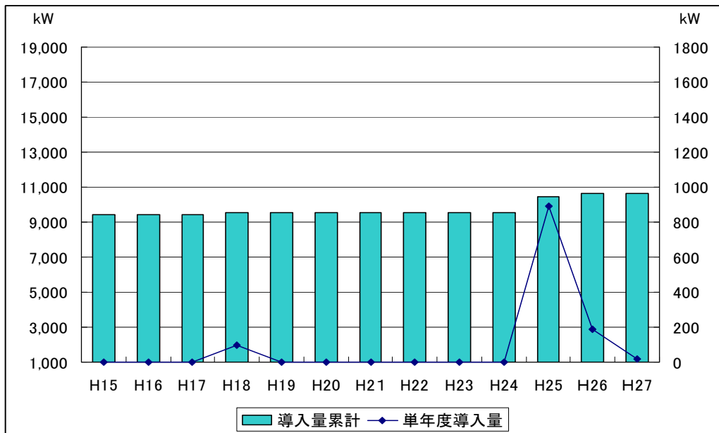
(図表 18) 本県の小水力発電の導入量の推移
