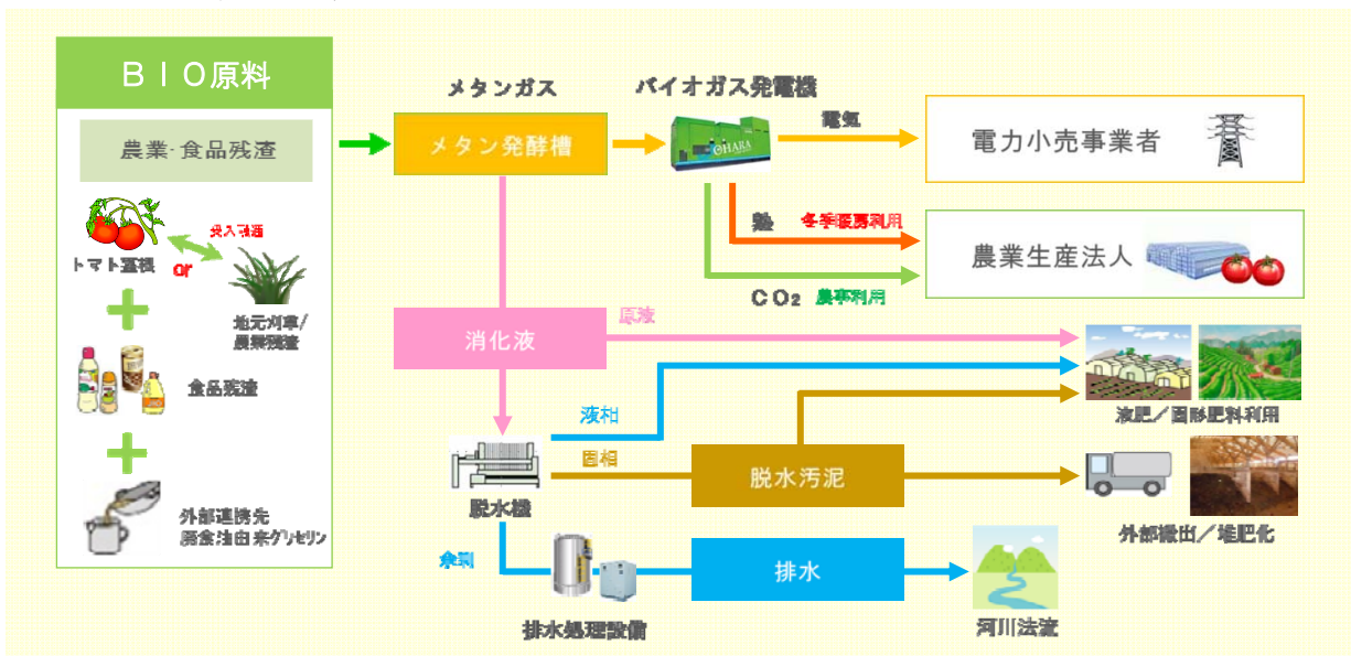
(図表 22) 農業生産法人等と連携したバイオガス発電所 (菊川市内)
