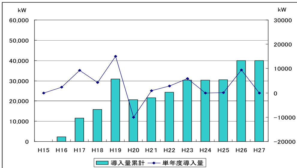
(図表 16) 本県のバイオマス発電の導入量の推移
