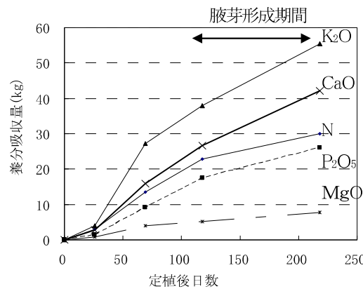
図3 プチパールの養分吸収経過 (静岡農林研)
