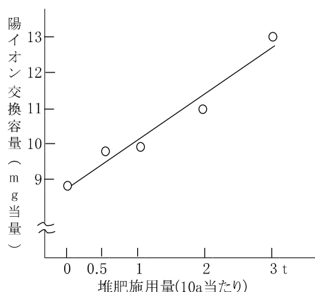
図1 堆肥施用量と陽イオン交換容量の関係 (高橋ほか)
