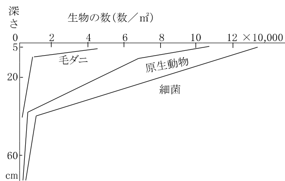
図2 土壌中での生物の分布
