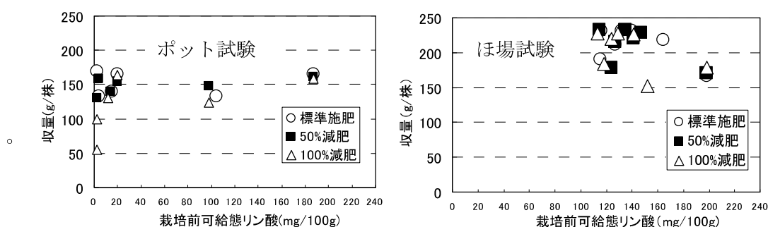
図 3 栽培前の可給態リン酸とチンゲンサイの収量
