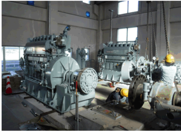
搬入された原動機（2台）
