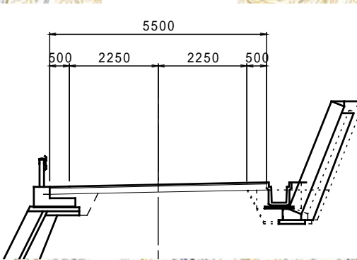
標準断面図
