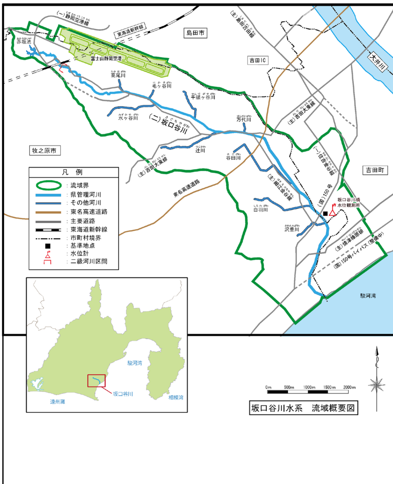
(参考図) 坂口谷川水系図
