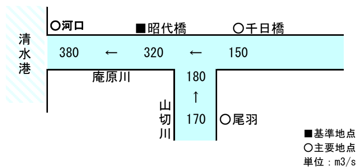
庵原川計画高水流量配分図
