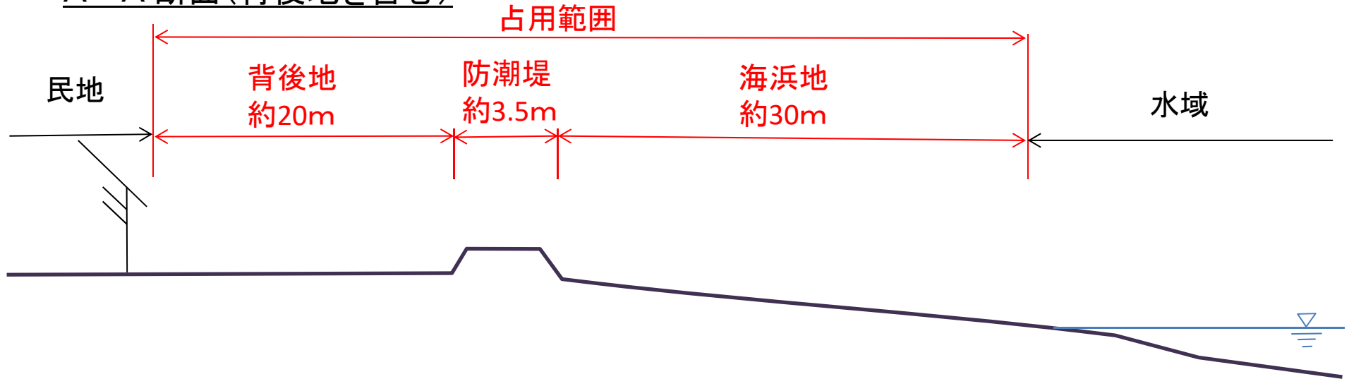
B-B'断面(背後地含まない)
