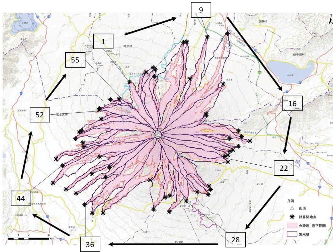
図 5.5-1 融雪型火山泥流のドリルマップ 計算開始点の配置一覧図
