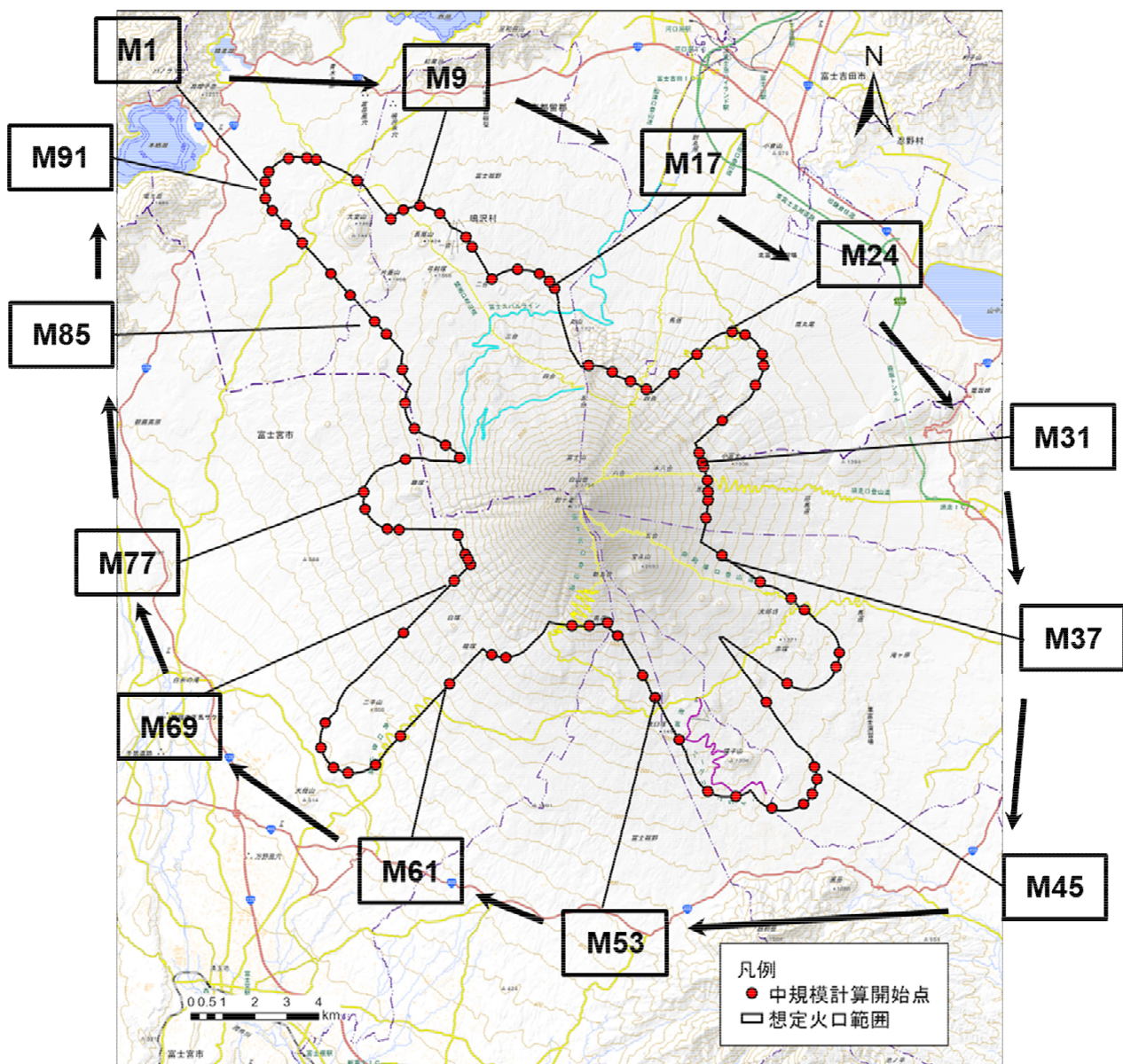
○ 中規模溶岩流のドリルマップ 計算開始点の配置一覧図（報告書_図 5.3-2）
