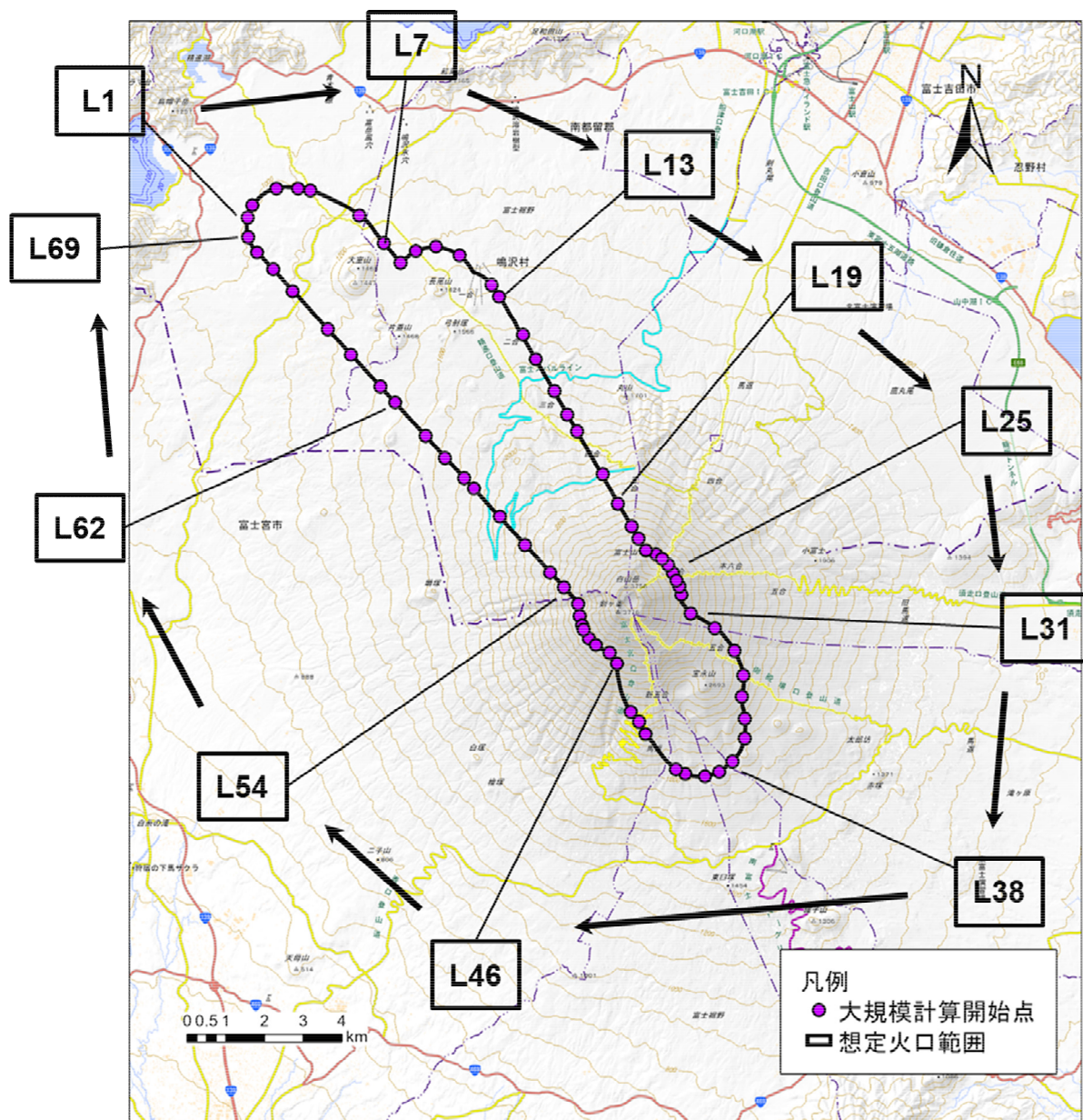
○ 大規模溶岩流のドリルマップ 計算開始点の配置一覧図（報告書_図 5.3-3）
