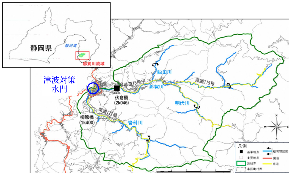
図 4-1 那賀川水系整備区間
