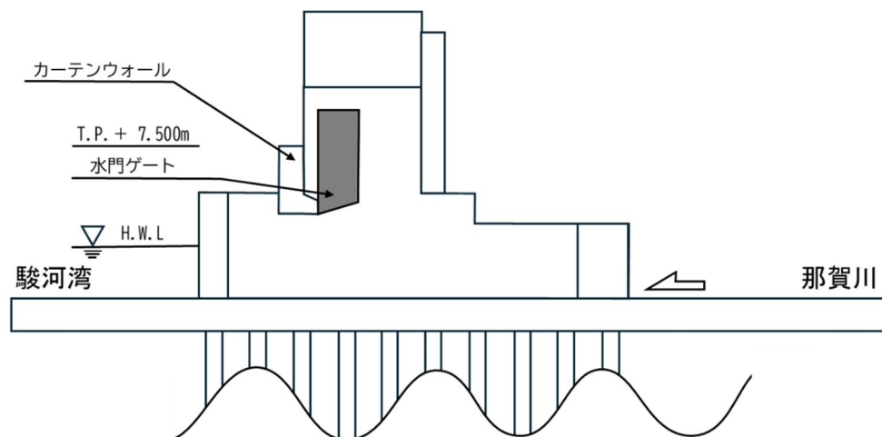
図 4-3 津波対策水門イメージ図（縦断図）
