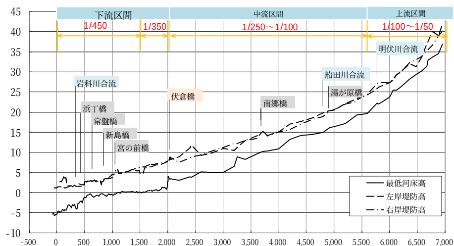
図 1-18 那賀川河道縦断面図
