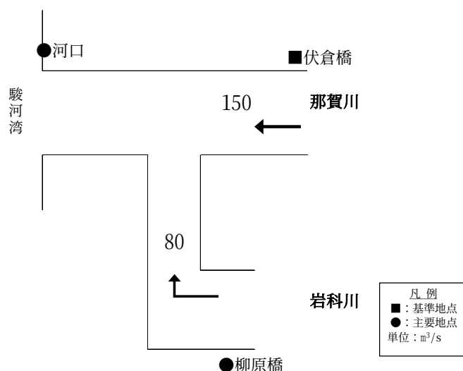
図 3-1 河川整備計画流量配分図
