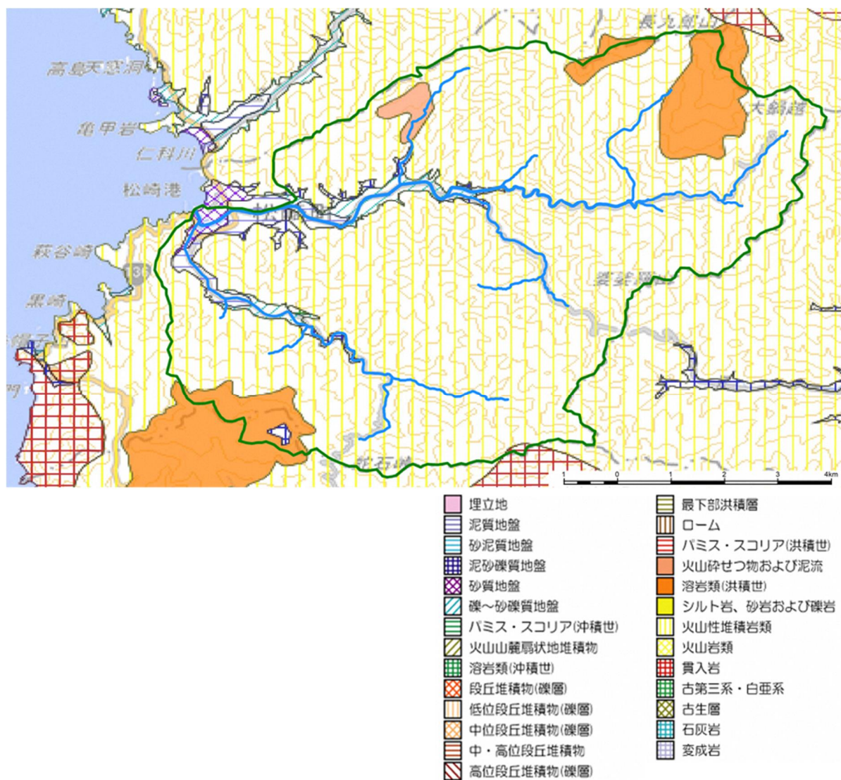
図 1-3 那賀川流域の地質図
