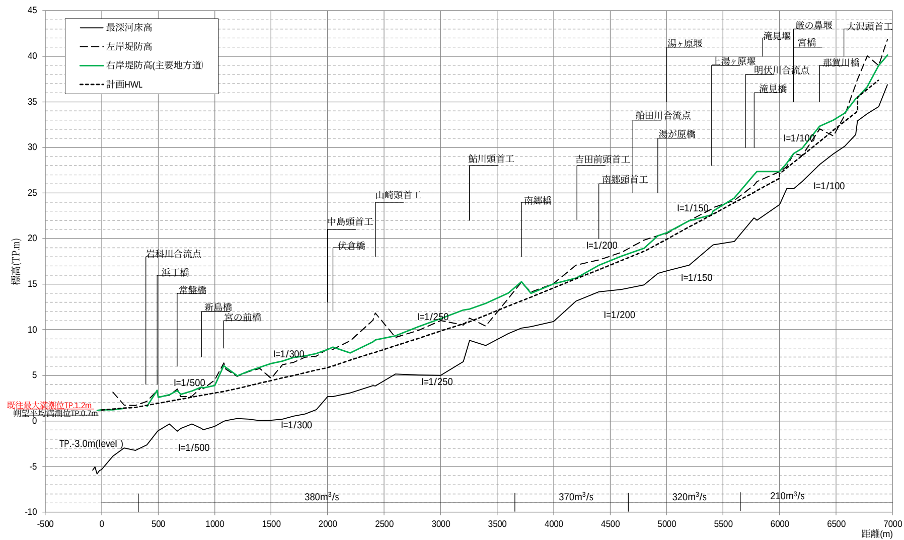
那賀川 縦断面図
