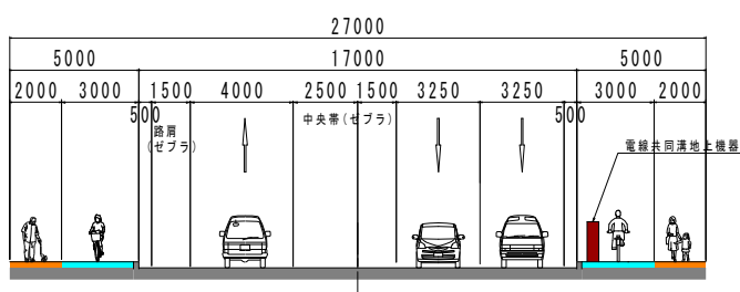
計画横断面図
