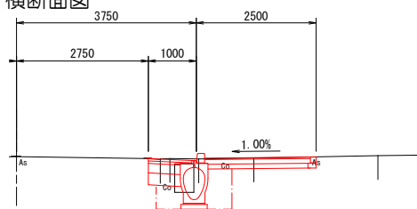
横断面図
