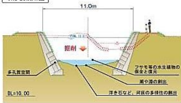
改修後横断面図
