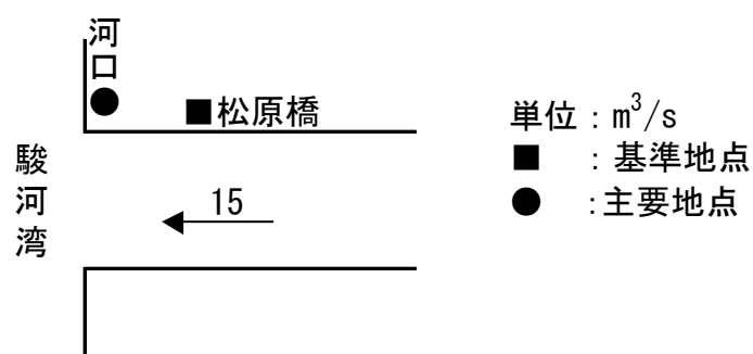
計画高水流量配分図
