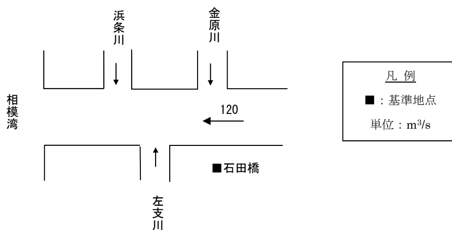
大賀茂川計画高水流量配分図
