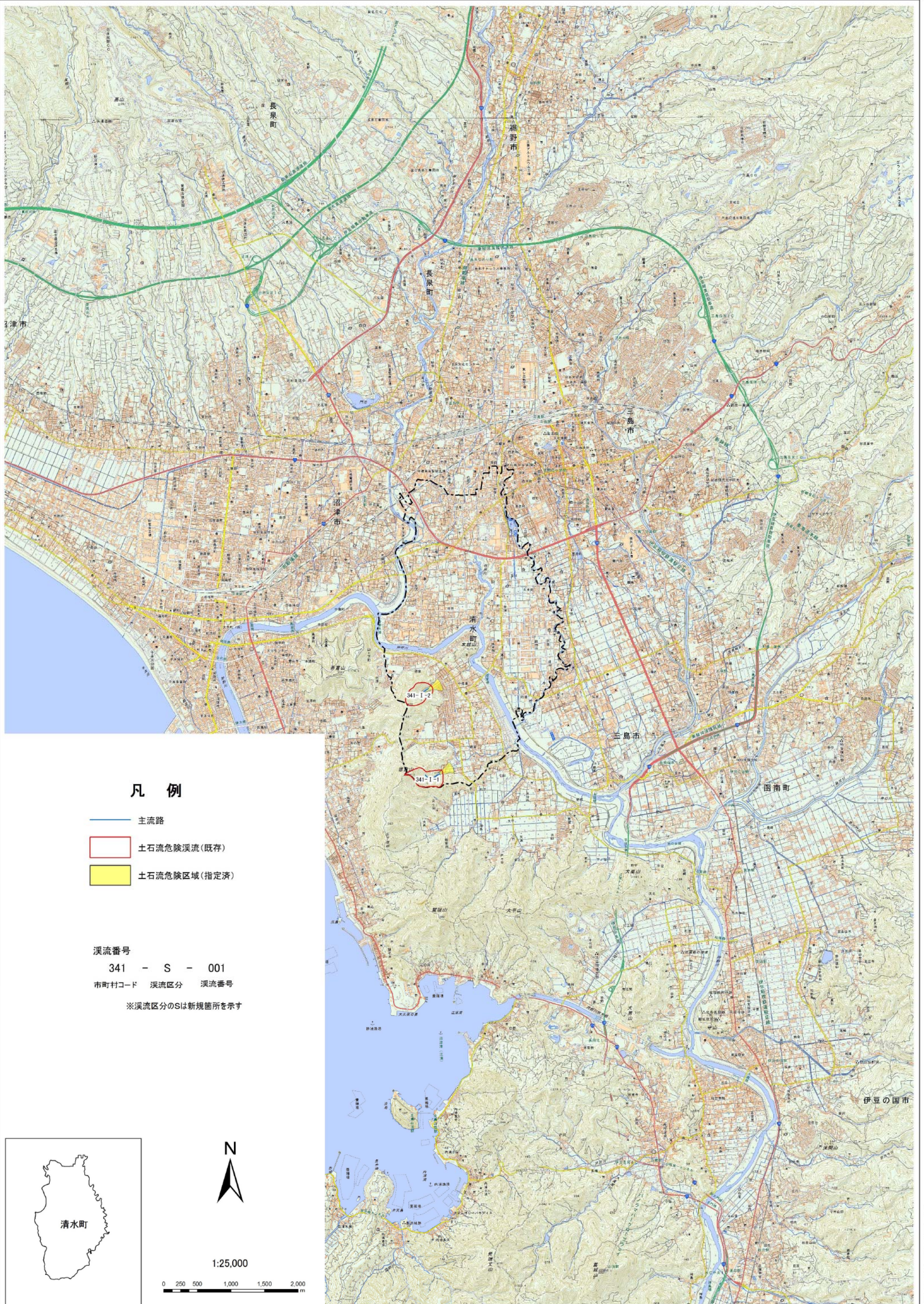
土石流抽出結果平面図(清水町)
