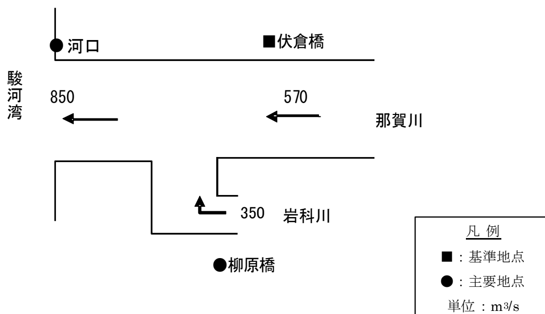
那賀川計画高水流量配分図
