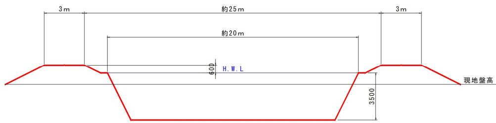
図 5-8 沼川新放水路標準断面図（築堤区間）
