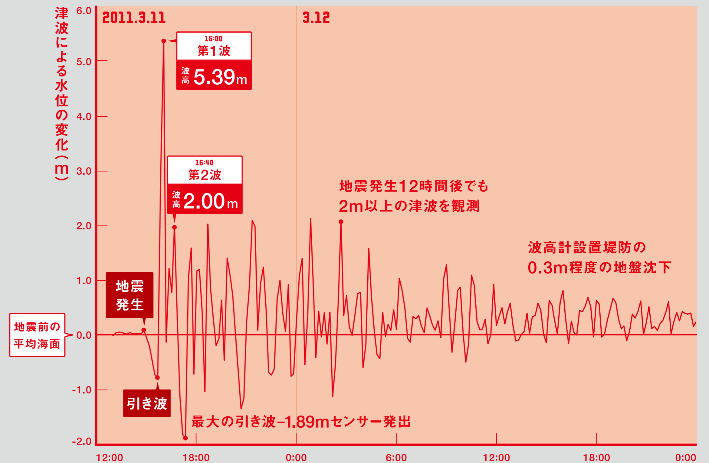
東北地方太平洋沖地震の 仙台湾での津波による水位変動データ
