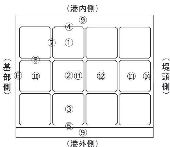
計算版数算出例
