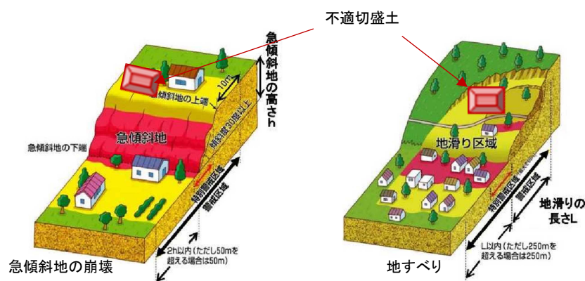
土砂災害警戒区域にある盛土のイメージ
