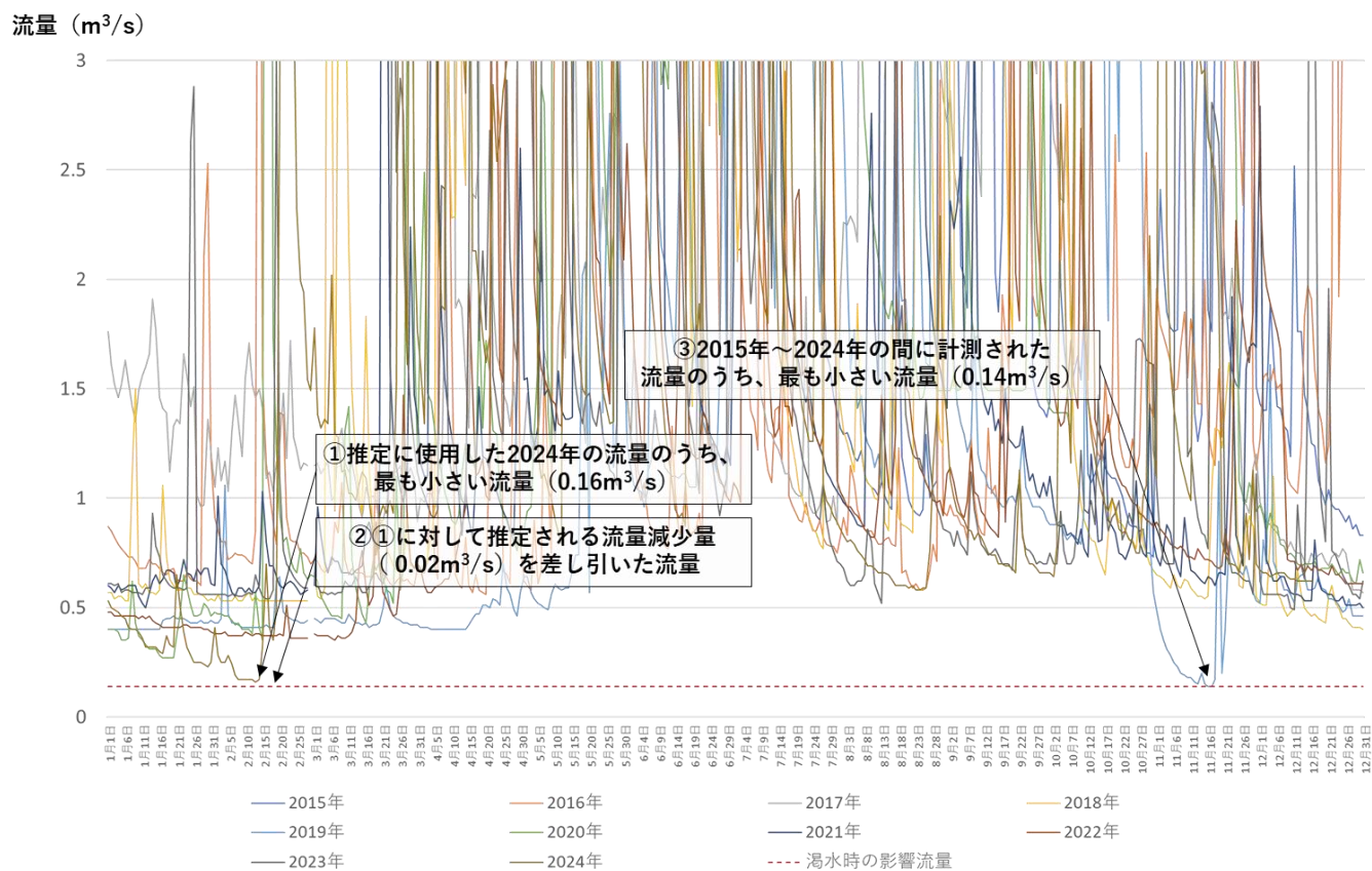
図 3 西俣地点に関する流量の整理
