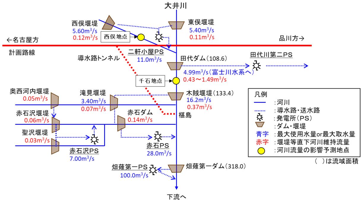
図2 大井川上流における利水の状況 2
