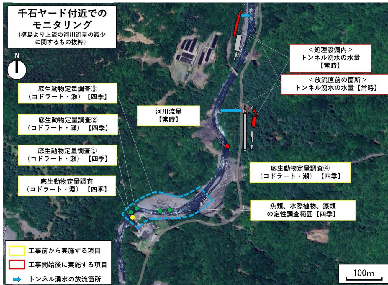
図 5 千石ヤード周辺における河川流量の変化に係るモニタリング計画
