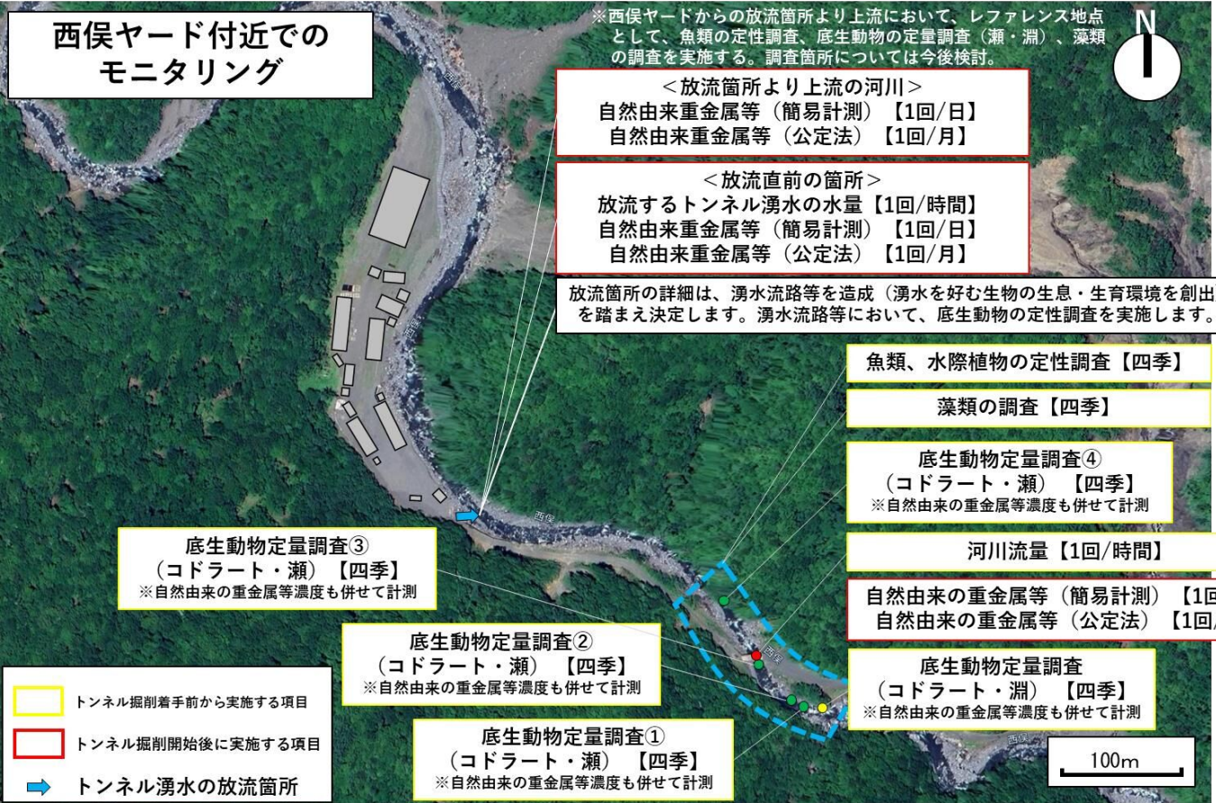
図 2 西俣ヤード周辺における自然由来重金属等に係るモニタリング計画
