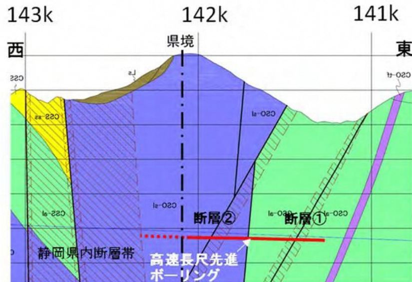
図 27 地質縦断図
