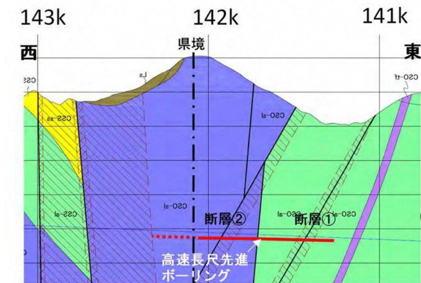
図 9 地質縦断図
