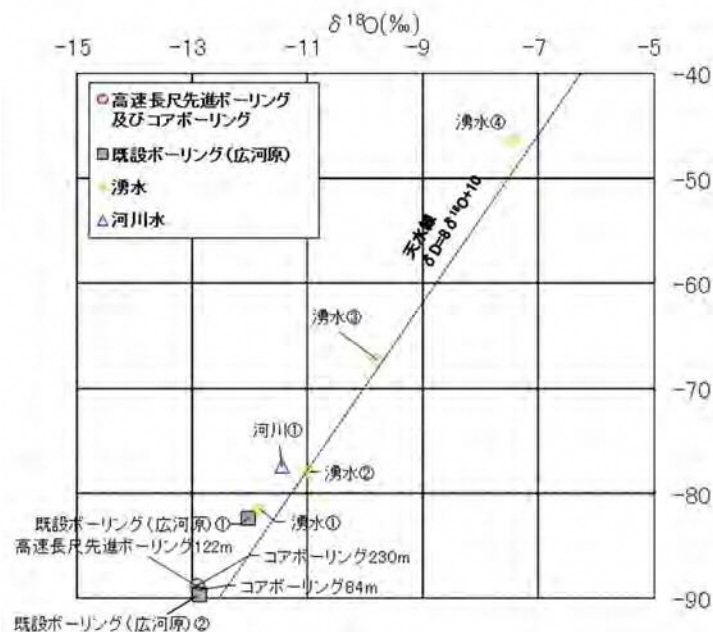
図 8 1 \delta ダイアグラムと Craig の天水線
