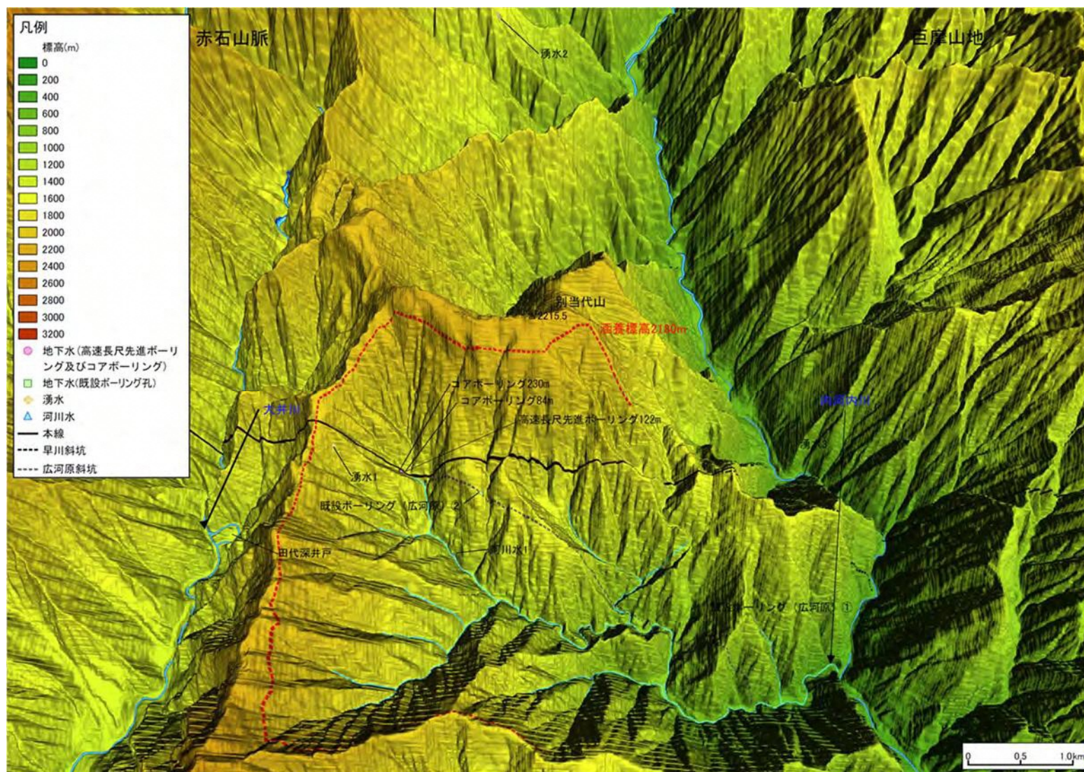
図 8 4 推定涵養標高線
