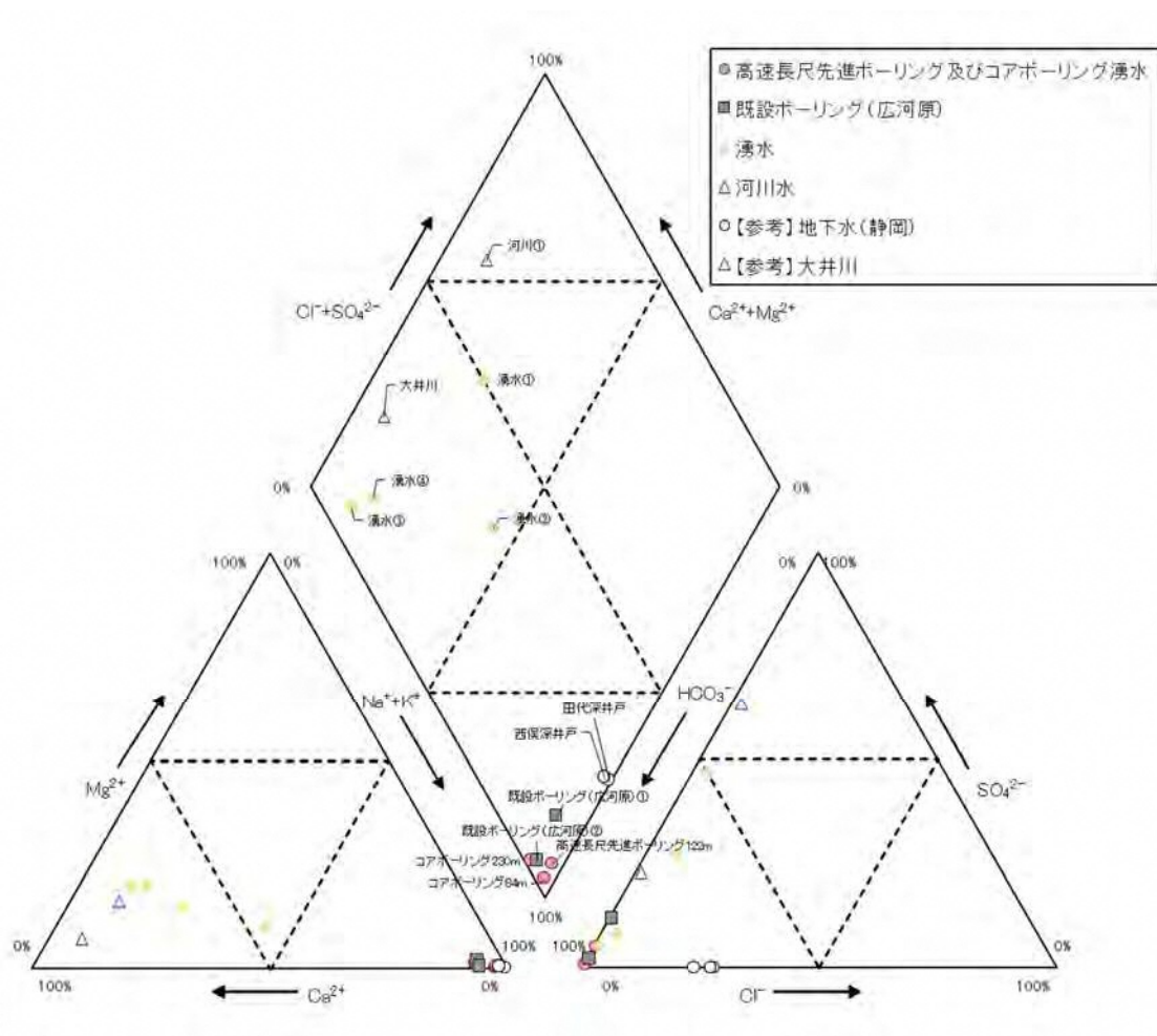
図 80 溶存イオン分析結果（水質組成図：トリリニアダイアグラム 8) ）
