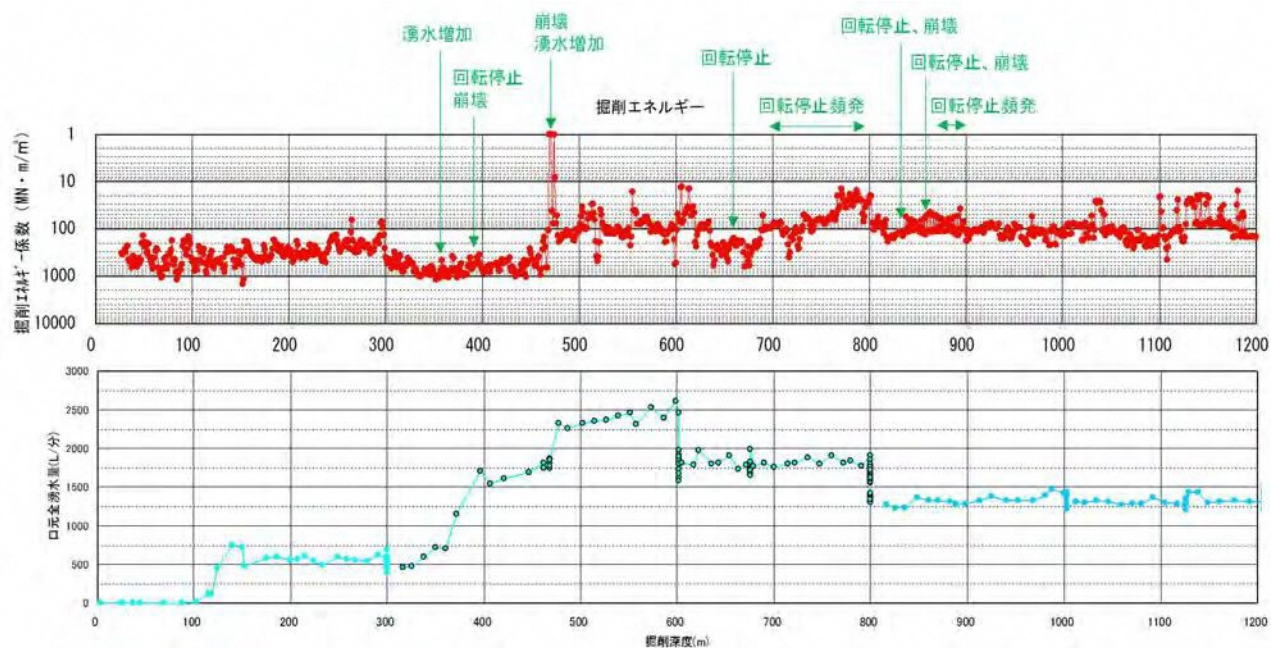
図 15 高速長尺先進ボーリングの調査結果
