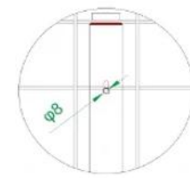
フックボルト取り付け詳細図 (S=2:1)
