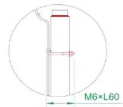
フックボルト取り付け詳細図 (S=2:1)
