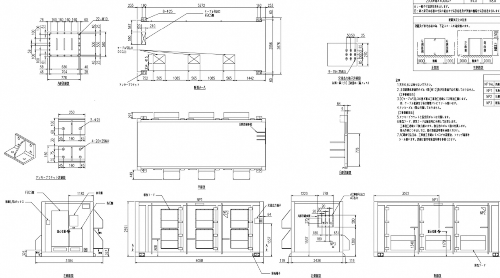
図 2-1-1 PCS コンテナ外形図 (標準仕様)
