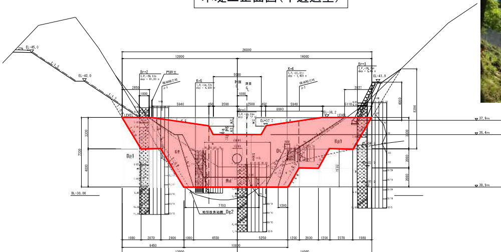
本堤工正面図(不透過型)
