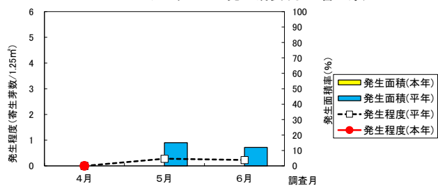
コミカンアブラムシの発生消長(小笠磐田原)
