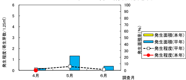
コミカンアブラムシの発生消長(川根地域)
