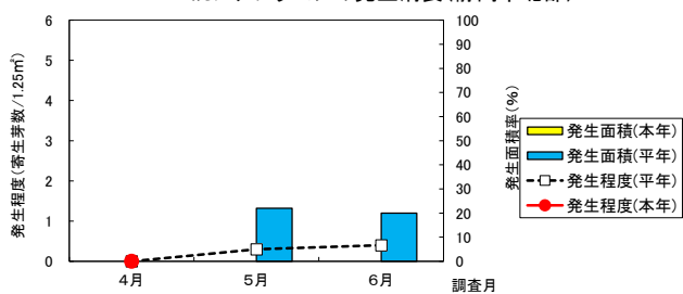
コミカンアブラムシの発生消長(静岡市北部)
