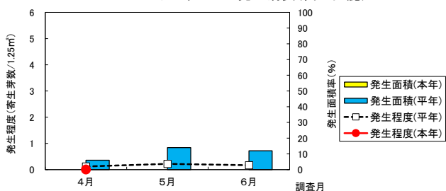
コミカンアブラムシの発生消長(富士山麓)
