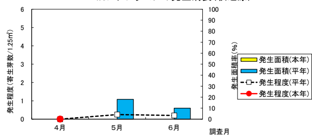
コミカンアブラムシの発生消長(牧之原)
