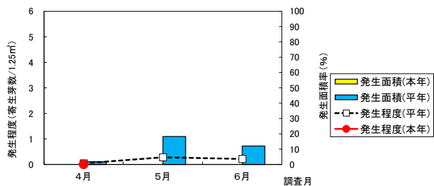
コミカンアブラムシの発生消長(県全体)
