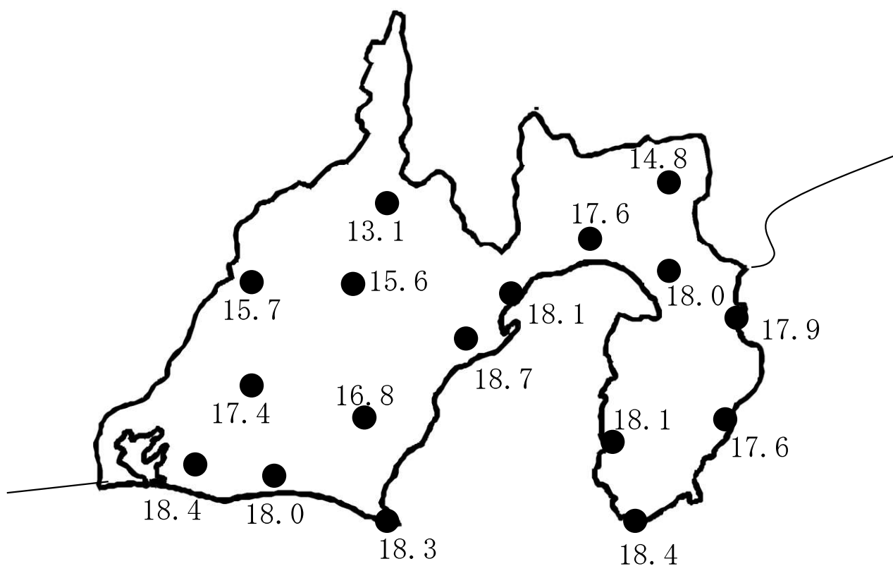
2024年静岡県内気象庁・アメダス年平均気温 (°C)
