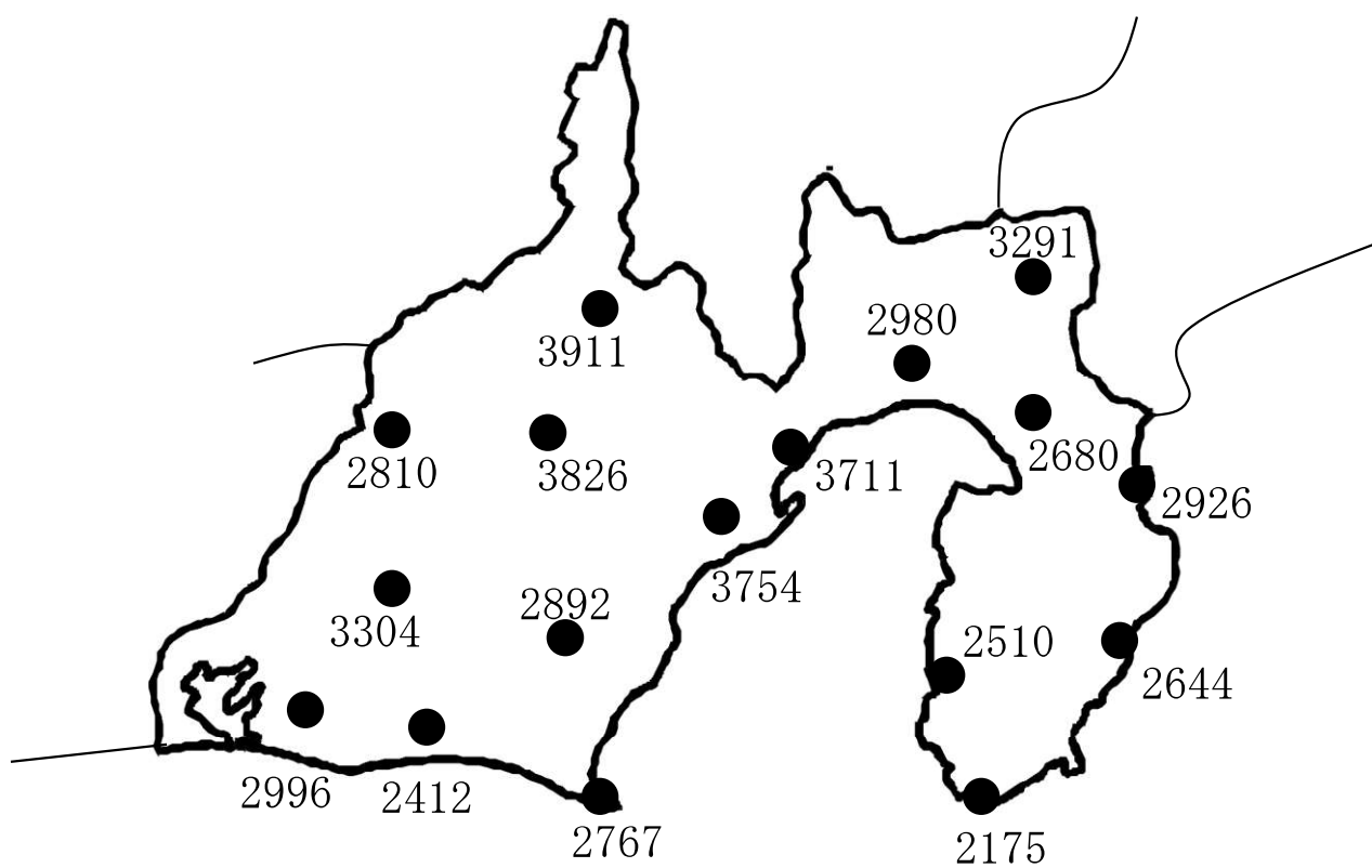
2024年静岡県内気象庁・アメダス年間降水量 (ミリ)
