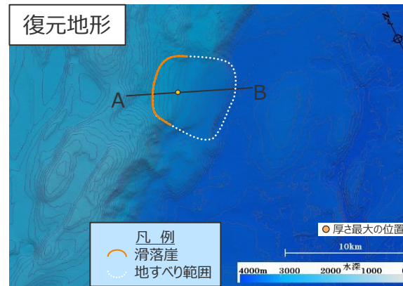
地すべり前の海底地形（復元地形）
