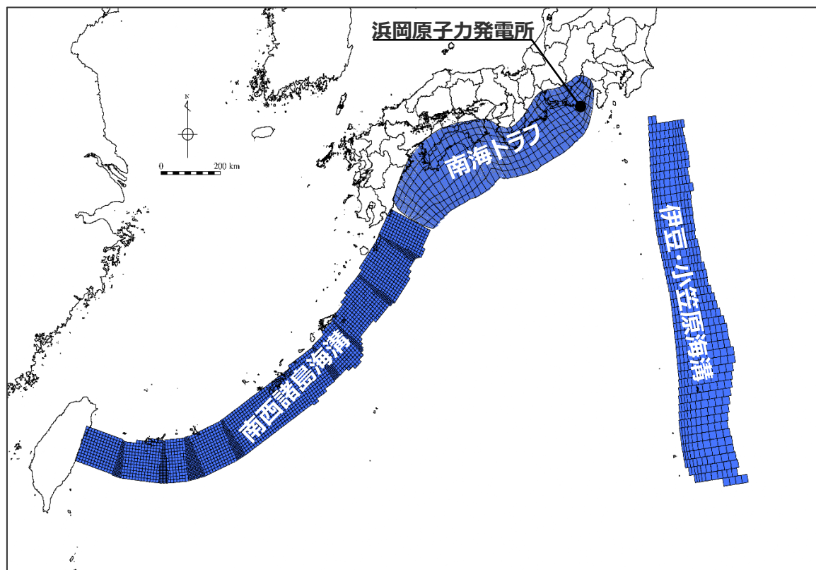
波源モデル
