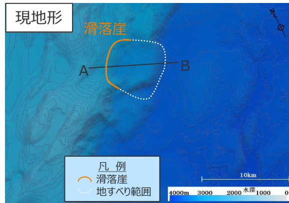
地すべり後の海底地形（現地形）
