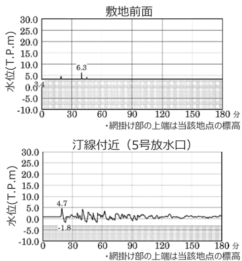
<水位の時刻歴波形>
