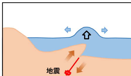
地震による津波
