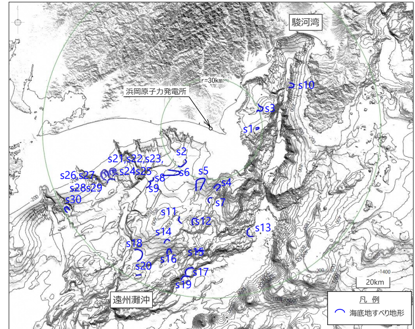
地形判読調査により抽出した海底地すべり地形の位置図
