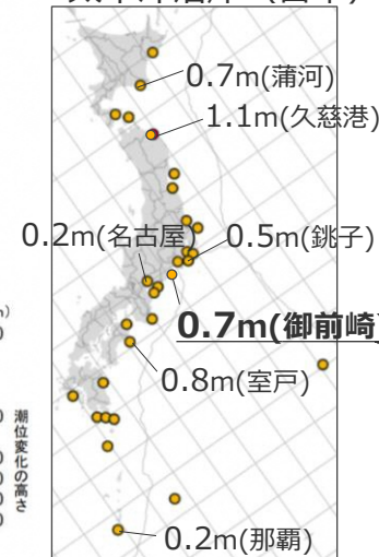
・数値は主な水位変動(場所) (気象庁(2022))
