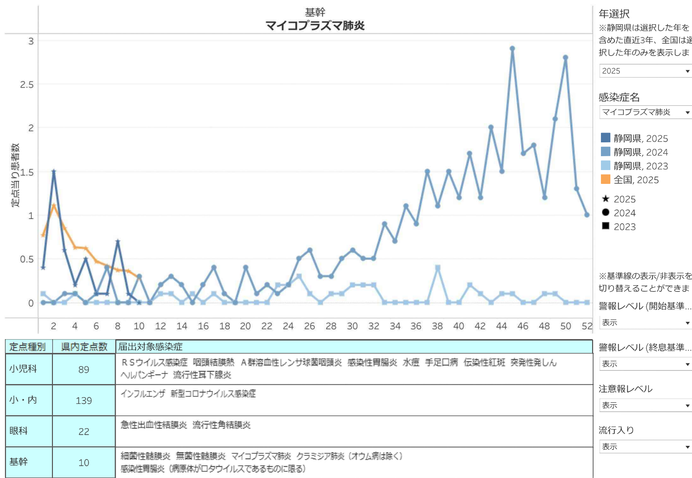
定点把握感染症推移 2025年 第10週までのデータに基づく
