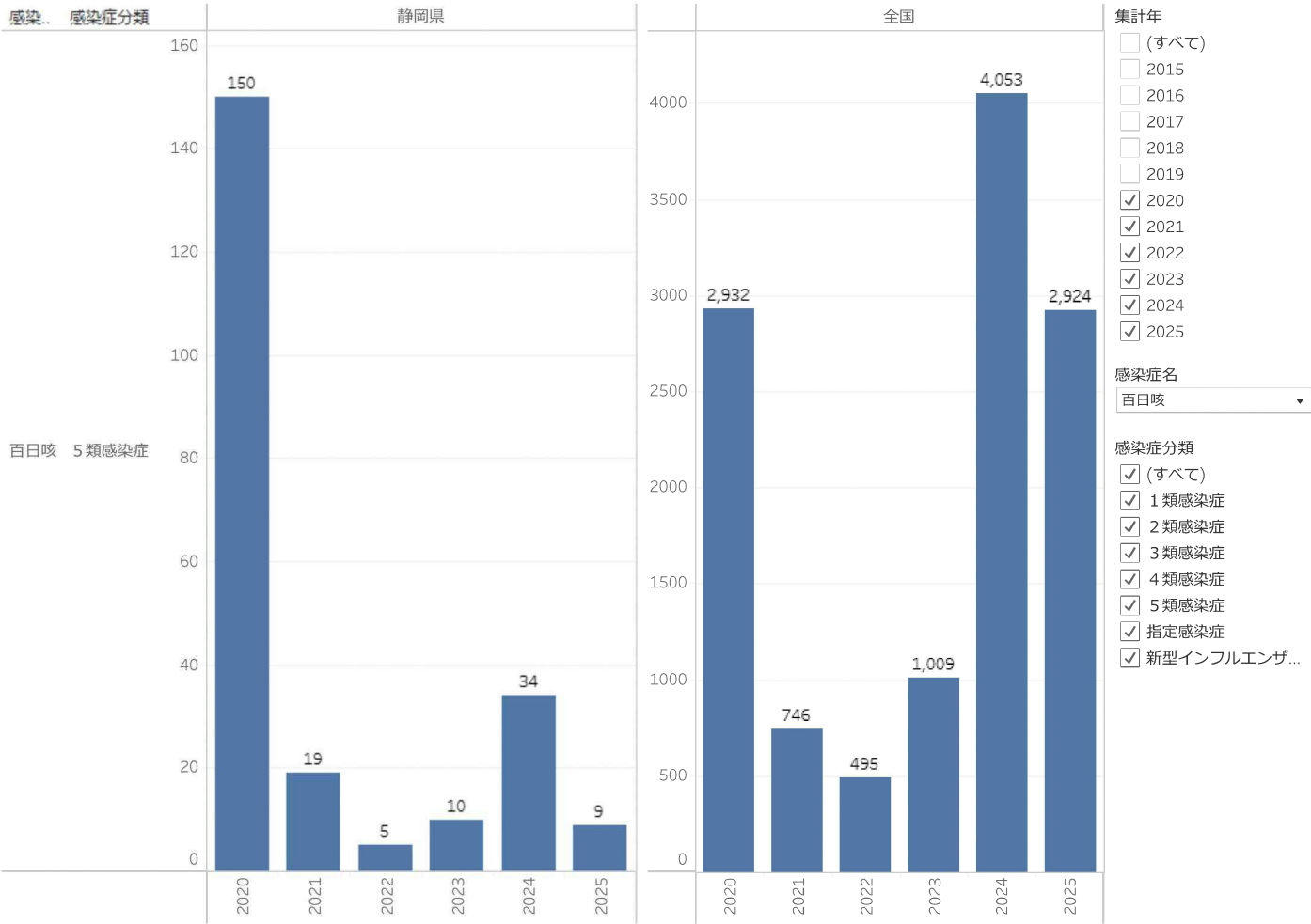
全数把握感染症年別累計
