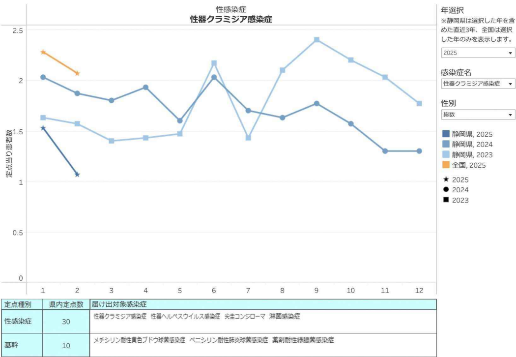
定点把握感染症(月報)推移グラフ 2025年02月までのデータに基づく
