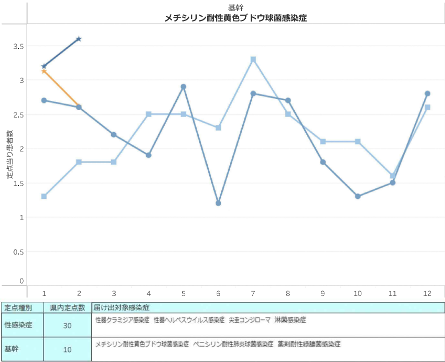
定点把握感染症(月報)推移グラフ 2025年02月までのデータに基づく
