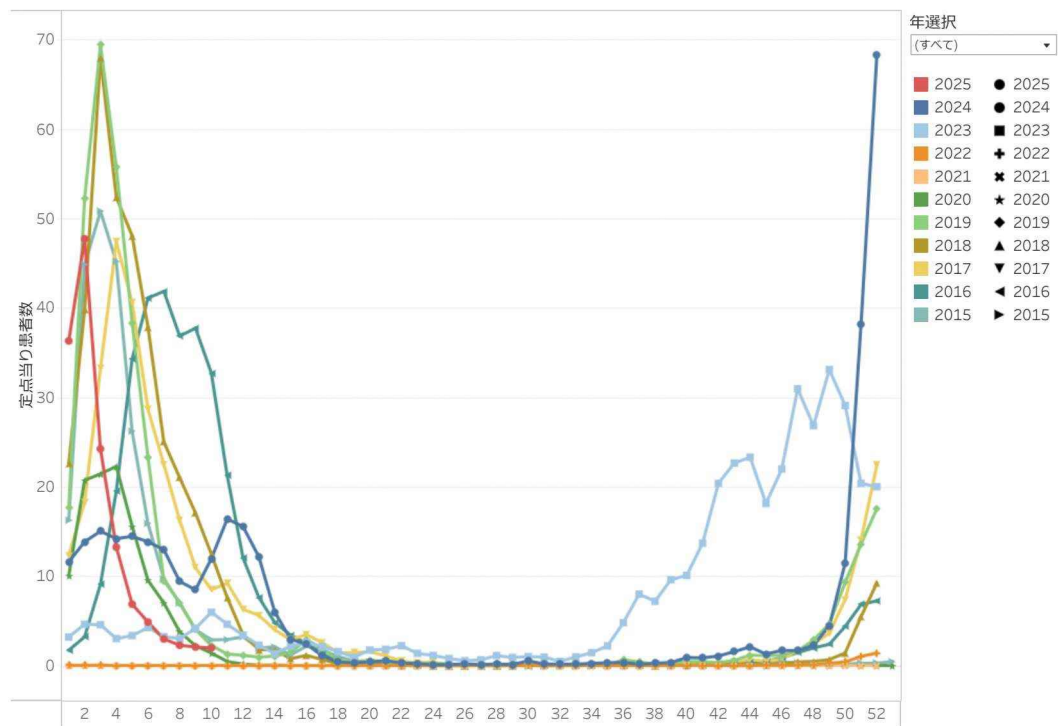
インフルエンザ報告者推移 2025年 第10週までのデータに基づく
