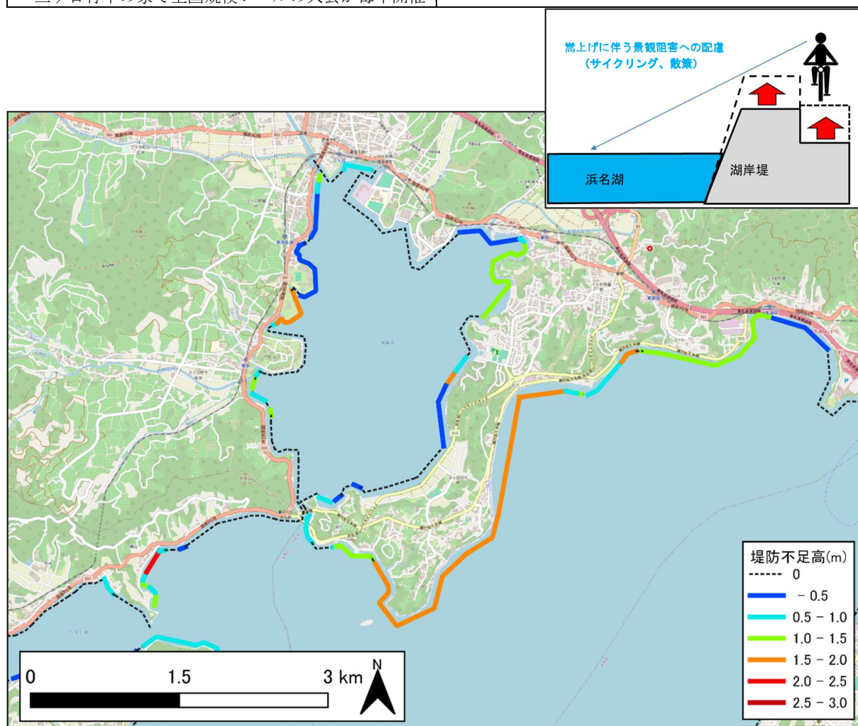
図 6.6 湖岸の防護目標に対する堤防の不足高（猪鼻湖エリア）
