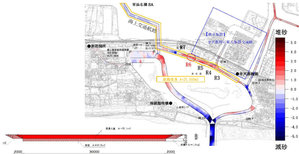
図 5.8 浜名湖航路改良事業 概要図
