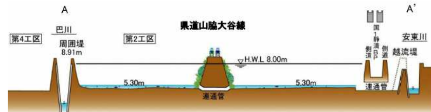
図 4-5 麻機遊水地第2工区横断イメージ図
