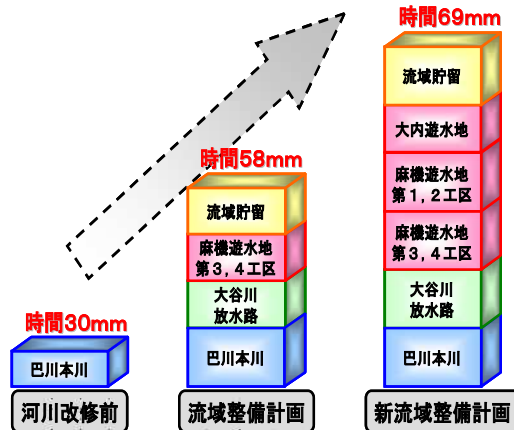
図 2-8 巴川流域の段階的な整備
