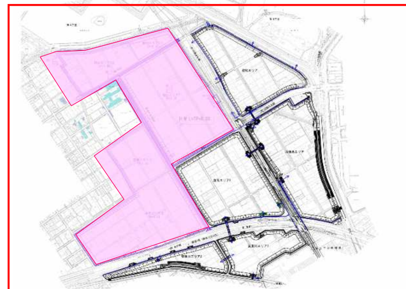
図 4-4 麻機遊水地第2工区平面図
