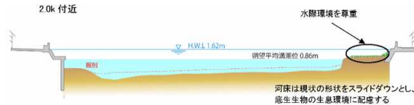
図 4-8 改修横断イメージ図
