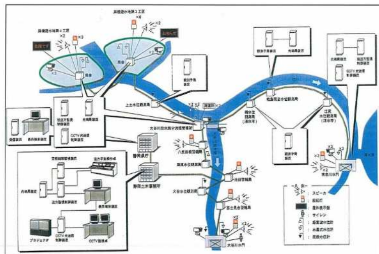
図2-11 巴川情報管理システム
