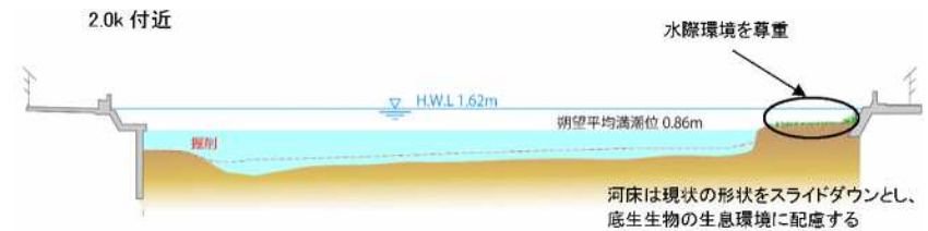
図 4-8 改修横断イメージ図
