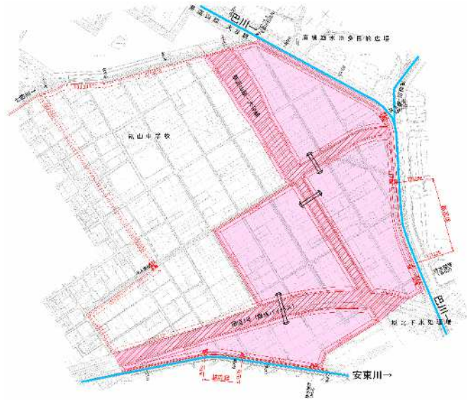
図 4-4 麻機遊水地第2工区平面図
