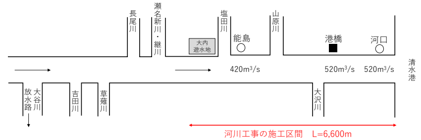
図 4-7 流量配分図
