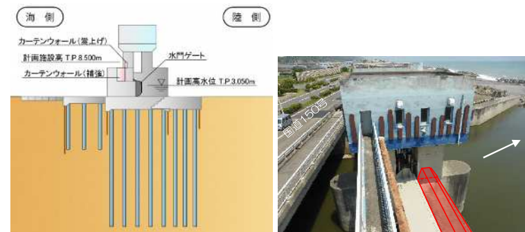
図 4-19 津波対策水門イメージ図
