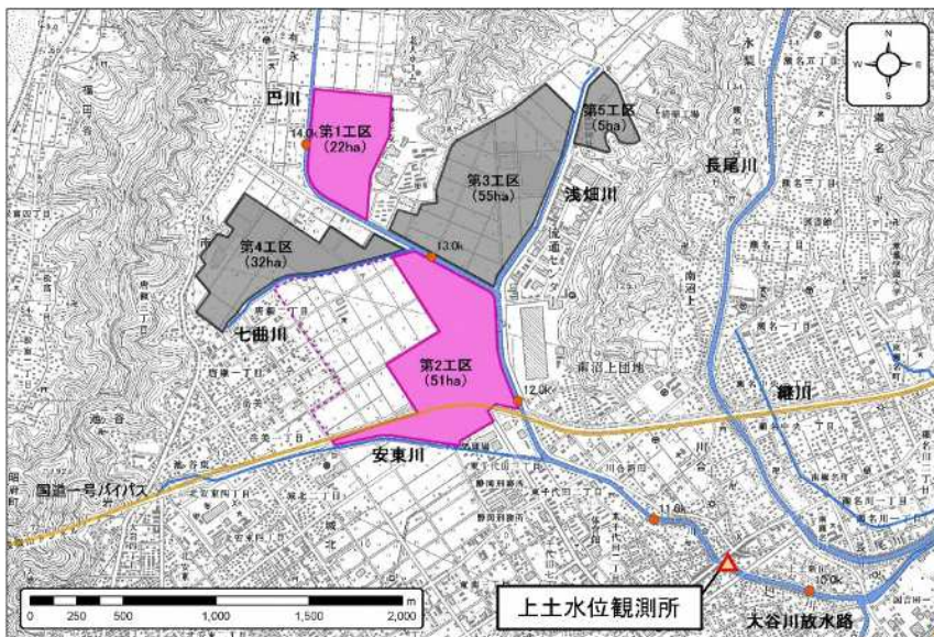
図 4-2 遊水地の整備箇所
