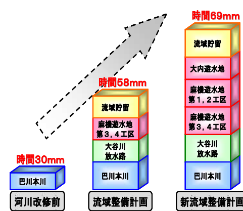
図 2-8 巴川流域の段階的な整備
