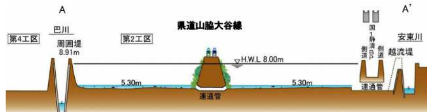
図 4-5 麻機遊水地第2工区横断イメージ図
