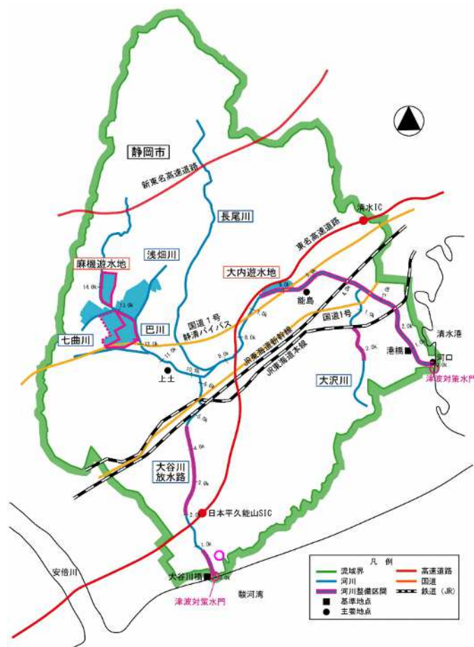
図 4-1 河川整備計画の主要な整備箇所
