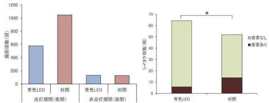
照明の有無によるキノコバエ類の防除効果 左: 飛来頭数、右: 被害頻度
