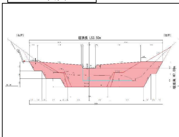
正面図
