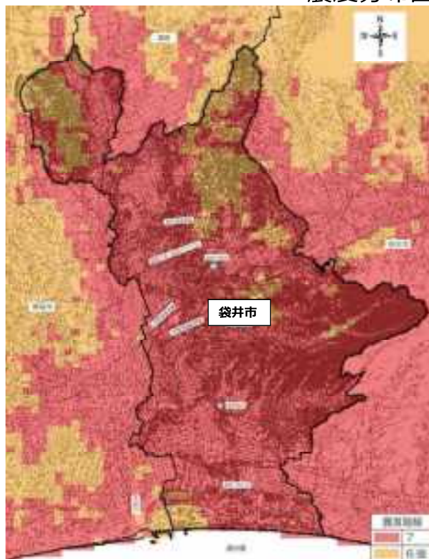
震度分布図
