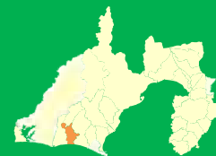
震度分布図
