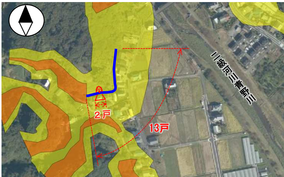
急傾斜地崩壊防止施設
