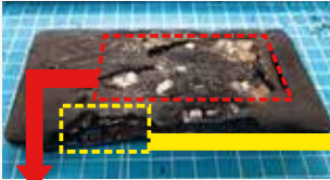
▲リチウムイオン電池部分の 背面カバーが大きく溶けている
